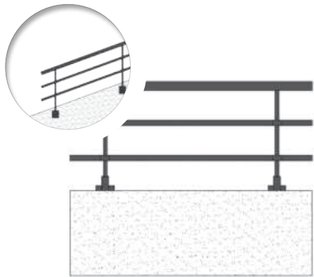
PAQUEBOT AVEC 2 TUBES DIAMÈTRE 30mm SUR MURET (HAUTEUR MINIMUM DU MURET 450mm)
