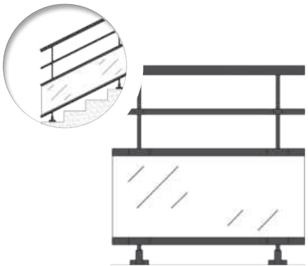
PAQUEBOT REPLISSAGE VERRE AVEC UN TUBE - DIAMÈTRE 30mm
