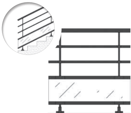
PAQUEBOT REPLISSAGE VERRE AVEC 2 TUBES - DIAMÈTRE 30mm
