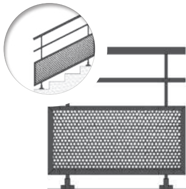
PAQUEBOT REPLISSAGE TÔLE PERFORÉE AVEC UN TUBE - DIAMÈTRE 30mm
