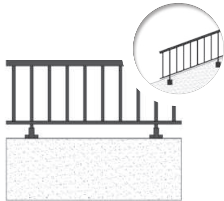
À BARREAUDAGE SUR MURET (HAUTEUR MINIMUM DU MURET 450mm)
